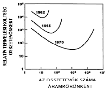
1. ábra A relatív termelési költség összetevőnként az összetevők áramkörönkénti számának függvényében
