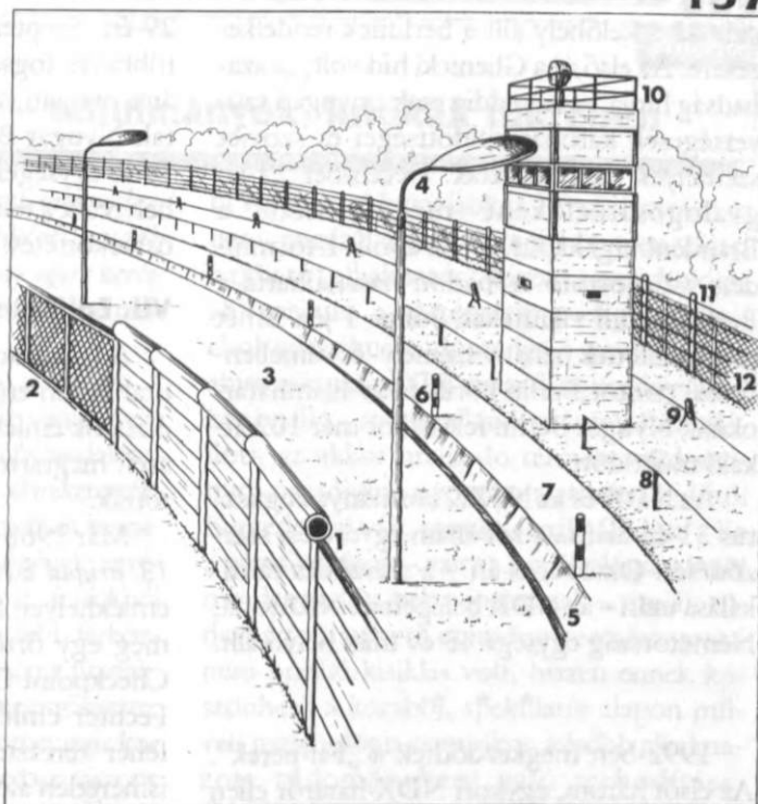
4. ábra. A BERLINI FAL SZERKEZETE
