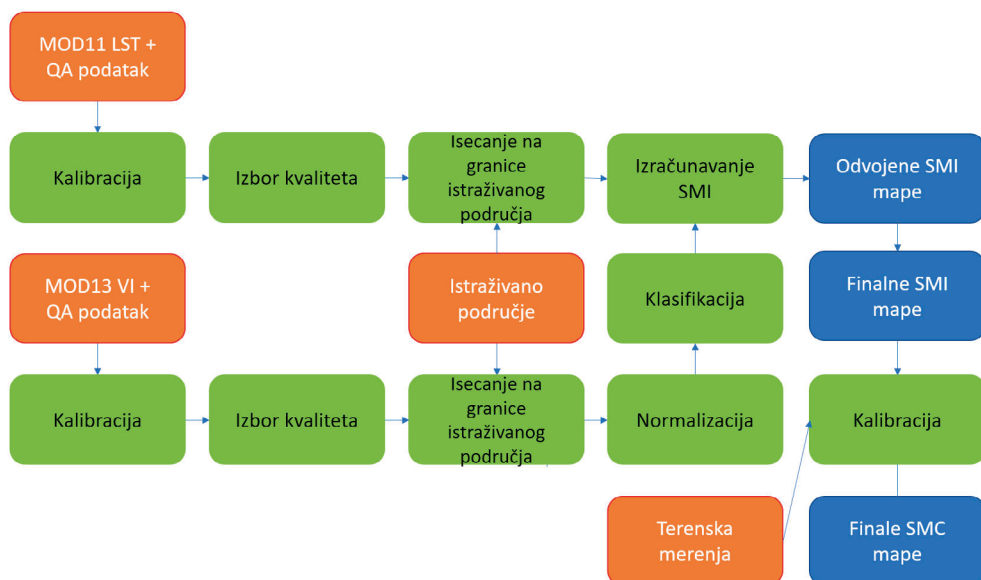
Slika 3.1. Proces obrade indeksa vlažnosti zemljišta
