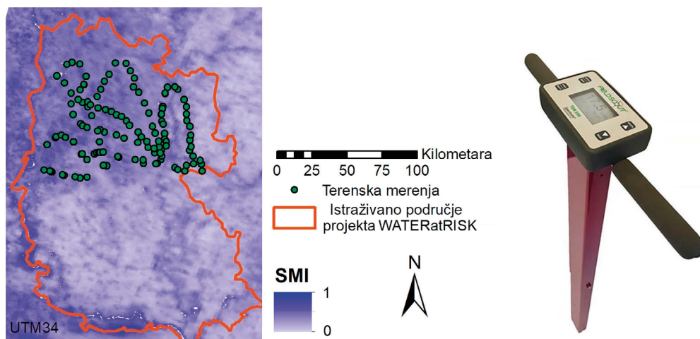
Slika 3.3. Serija terenskih merenja 27. marta 2019., kao i instrument za merenje FieldScout TDR350
