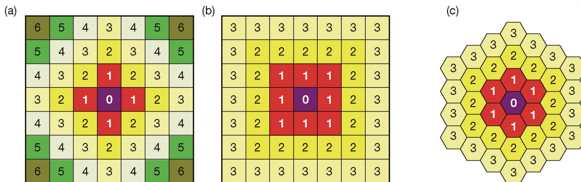
7. ábra: Kohonen modellezés alapján a neuronok legközelebbi szomszédai (4-6-8) [11] Figure 7: Closest neighbors of the neurons based on Kohonen modeling (4-6-8) [11]
