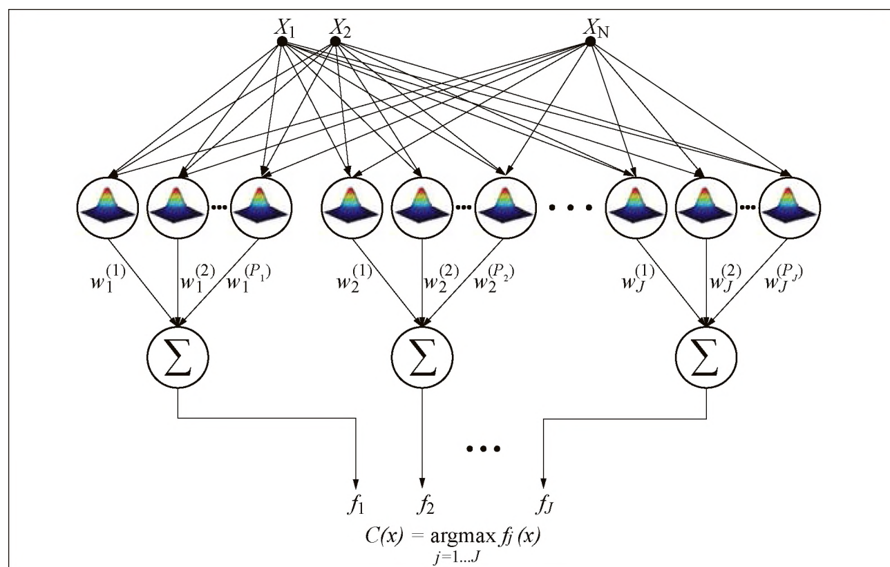
9. ábra: Valószínűségi neurális hálózat (PRNN) sematikus ábrája [32] Figure 9: Schematic representation of the Probabilistic Neural Net (PRNN) [32]
