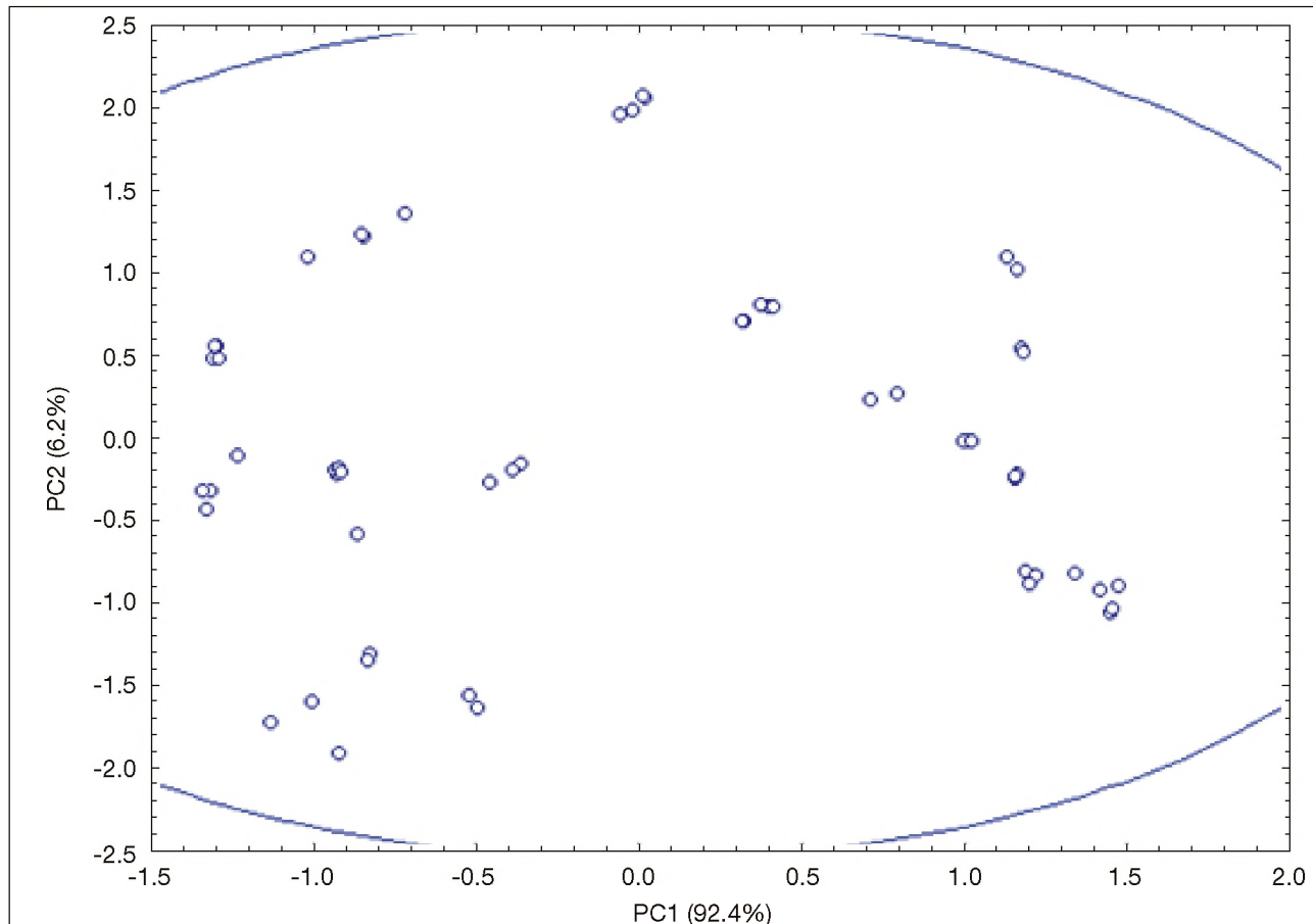
6. ábra: A PCA elemzés eredménye
