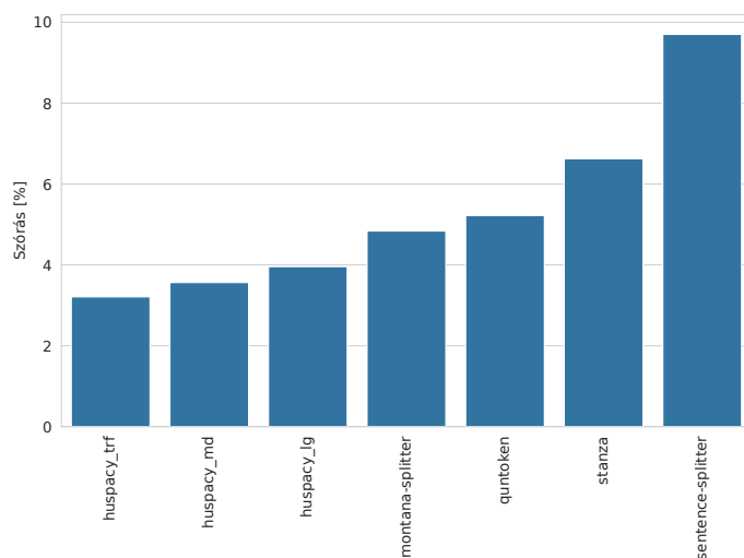
2. ábra: Az egyes szegmentálási megoldások doméntól való függése, Szeged Treebank F_1 értékek szórása
