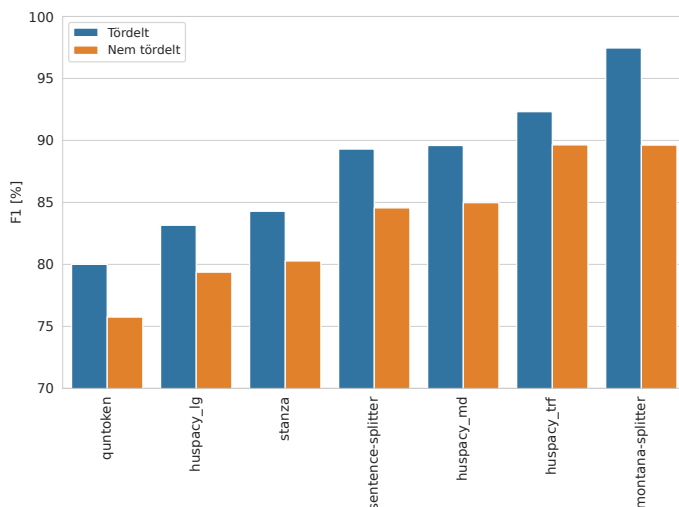
3. ábra: Mondatszegmentálók F_1 értékének tördeléstől való függése
