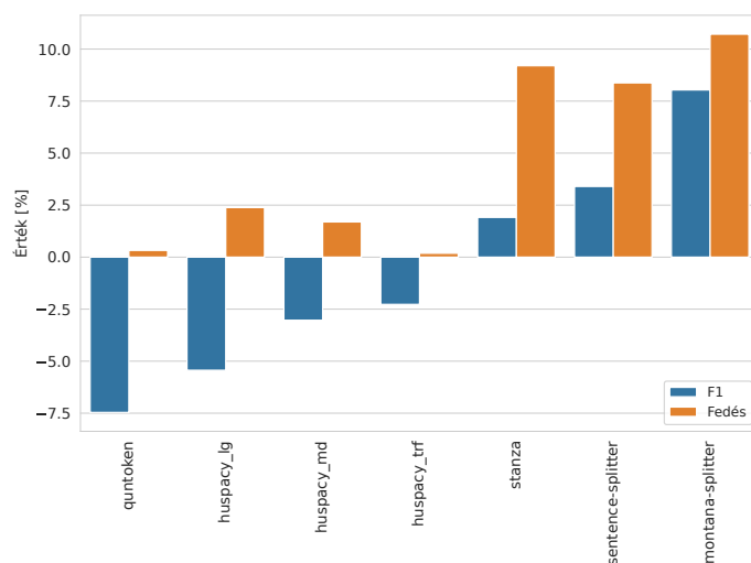
1. ábra: Az egyes szegmentálási megoldások aldoméntól való függése, a HuCoDe és a Szeged Treebank jogi alkorpusza közti különbség, fedés és F_1 értékben
