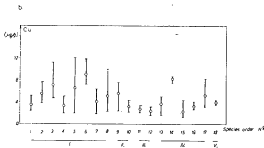
b) Cu
