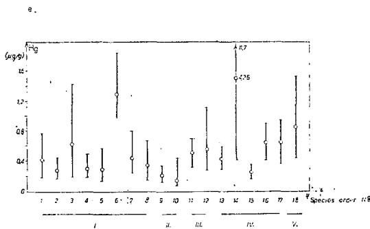
e) Hg
